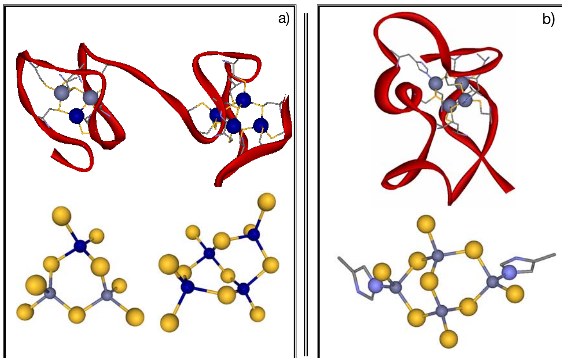
Figura 2.- Estructures tridimensionals, resoltes per RMN, de MTs enllaçades a ions divalents: a) Zn_2Cd_5 -MT2 de mamífer (rata) resolta per difracció de raigs X i els seus dominis \beta i \alpha formats pels agregats Cd_1Zn_2-(SCys)_9 i Cd_4-(SCys)_{11} , respectivament i b) Zn_4 -SmtA de cianobacteri (MT de Synechococcus ) i l'agregat Zn_4-(SCys)_9(NHis)_2 que forma.
